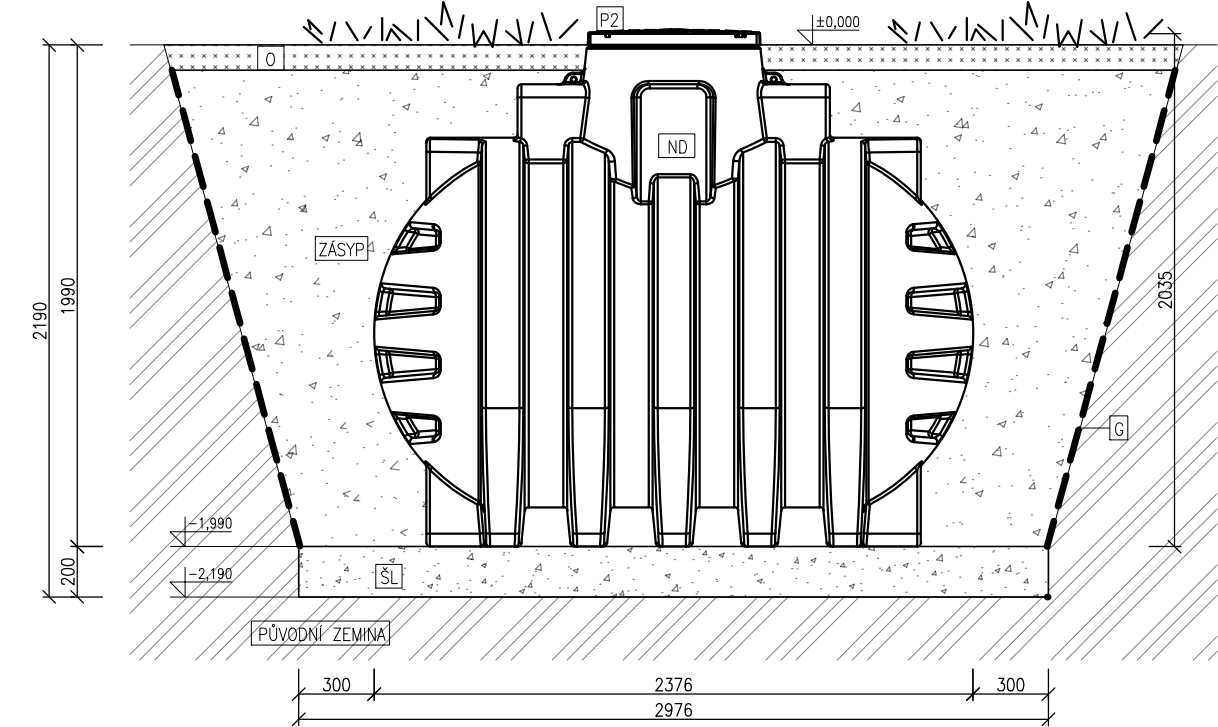
ŘEZ
