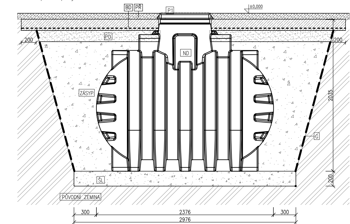
ŘEZ
